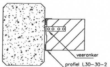
AANSLUITING AAN BETON-KOLOM OF-WAND
