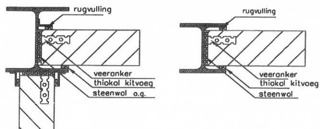
AANSLUITINGEN AAN STALEN KOLOMMEN
