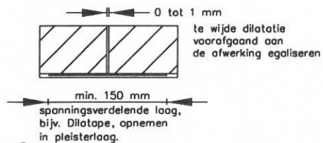
⑤ KOUDE DILATATIEVOEG
