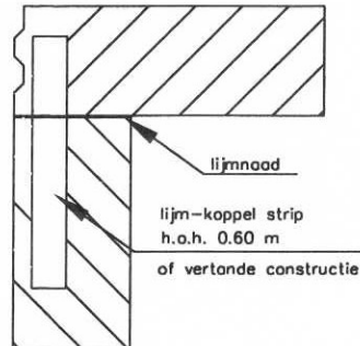
③ WAND-AANSLUITING
