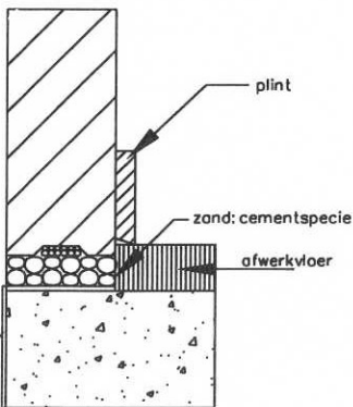
② VLOER-AANSLUITING
